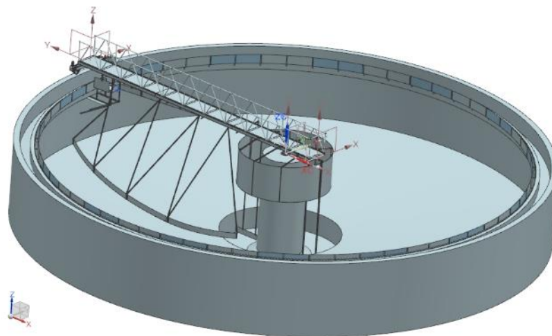
оборудование для радиальных отстойников
